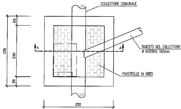
PIANTA
