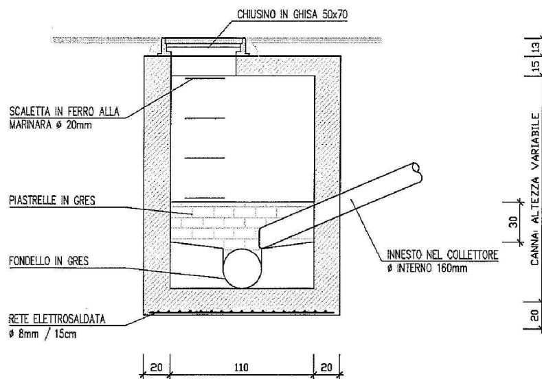
SEZIONE A-A
