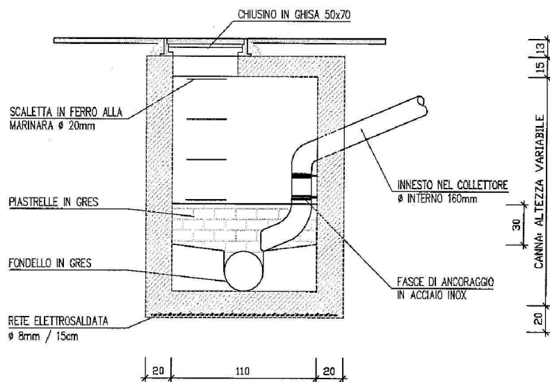
SEZIONE A-A
