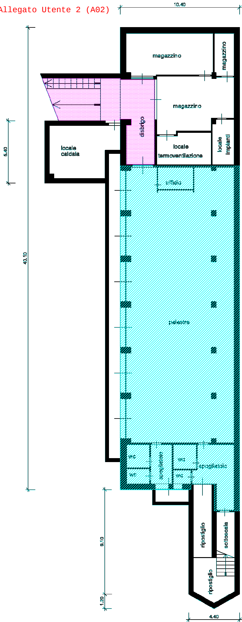
PIANTA PIANO SOTTOSTRADA
