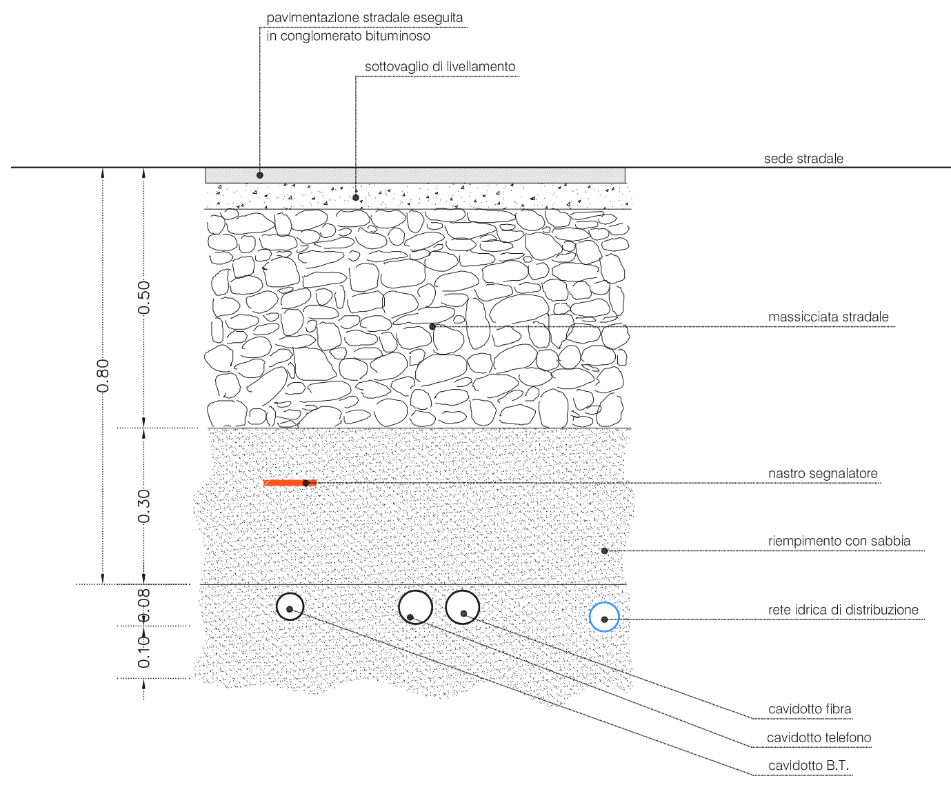
PARTICOLARE SCAVO SOTTOSERVIZI -scala 1: 10-
